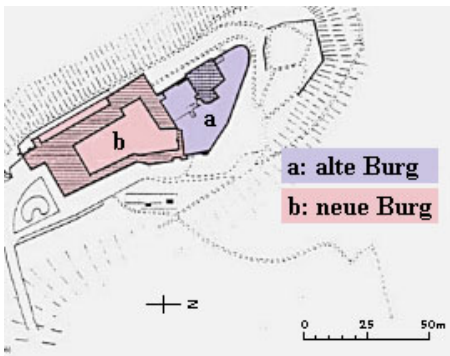
Lage der alten und neuen Burg auf aktuellem Grundrissplan
